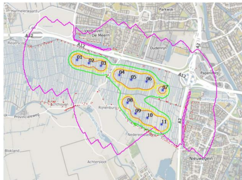
Geluidcontouren en invloedsgebied slagschaduw voor de voorbeelduitwerking van de visie. Dit is voor de woonwijken de worst case situatie. Legenda: ■ L dsn 45 dB ■ L dsn 47 dB ■ L dsn 41 dB ■ Invloedsgebied slagschaduw
